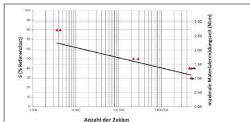
Wöhlerlinie
