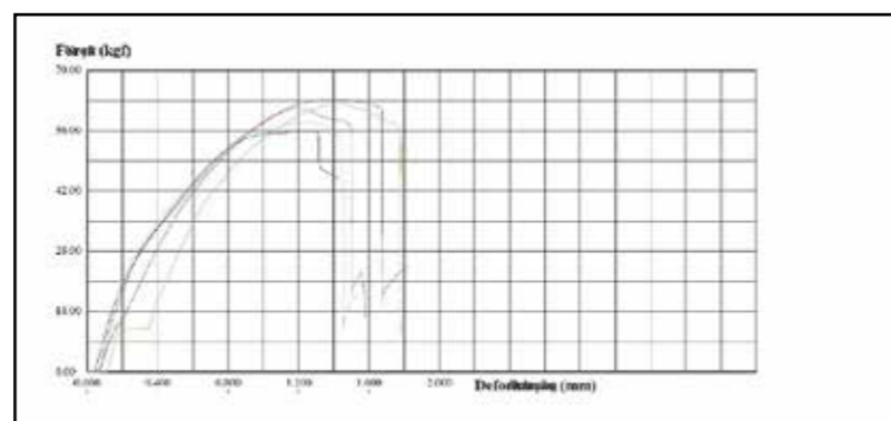
Kurvenverlauf während der statischen Belastungsprüfung
