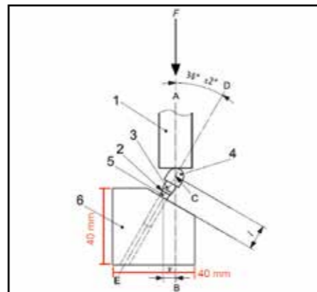
Darstellung des Testaufbaus
